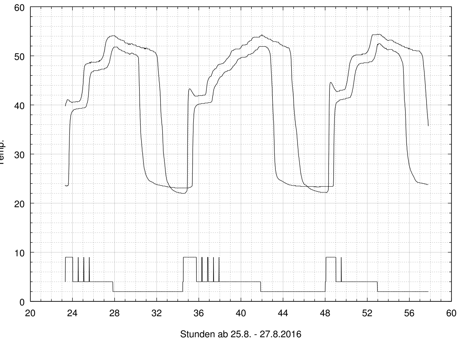
Kompr. & Temps: Fuehlerorte ganz unten und zweitunterst
